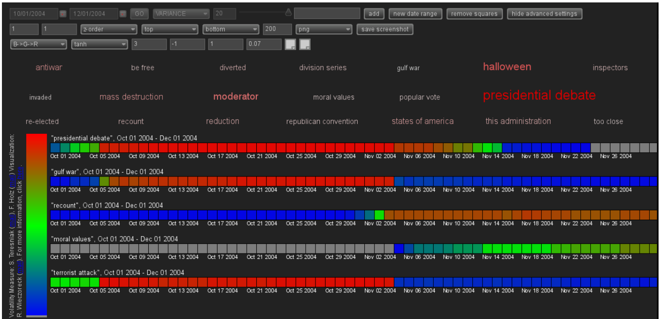
Abb. 6: Der Zeitraum um die US-Präsidentschaftswahl am 2.11.2004. Terroristische Angriffe ( terrorist attack ) wurden im Wahlkampf mehrfach thematisiert. Der starke Anstieg der Kontextvolatilität dieses Terms korreliert im Zeitraum nicht mit der Termfrequenz.
