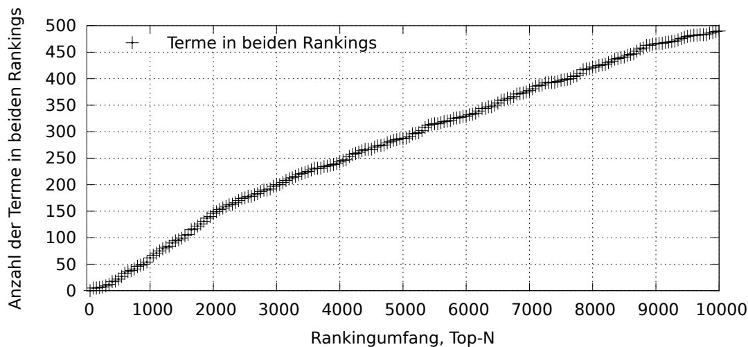
Abb. 2: Anteil der Terme, die in beiden Rankings – tf-idf und Kontextvolatilität – vorkommen, in Abhängigkeit vom Rankingumfang. Im Mittel lässt sich knapp jedes 20. Wort in beiden Rankings finden.
